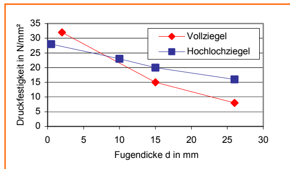
Bild 1: Einfluss der Lagerfugendicke d_F auf die Mauerwerkdruckfestigkeit \beta_{D,mw} nach [1]
