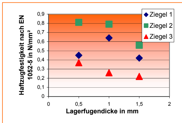
Bild 2: Verbundfestigkeit in Abhängigkeit von der Fugendicke
