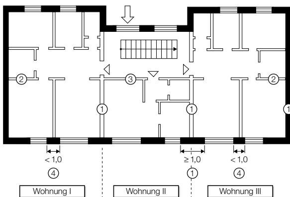
Bild 2 Benennung von Bauteilen nach DIN 4102
